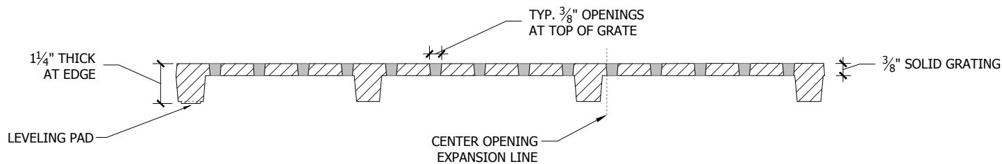
Section A-A'
