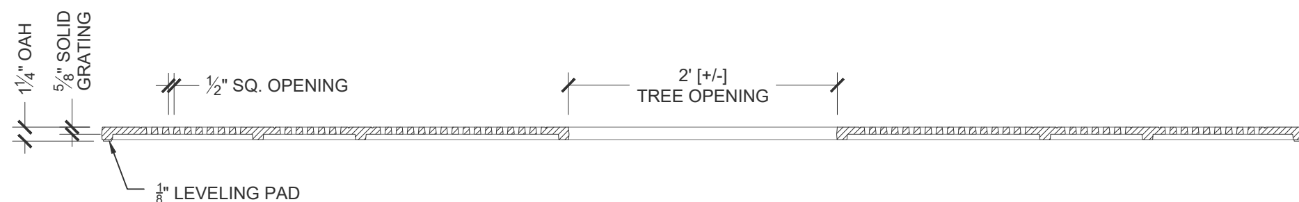
Cross Section Scale: 1" = 1' 0"
