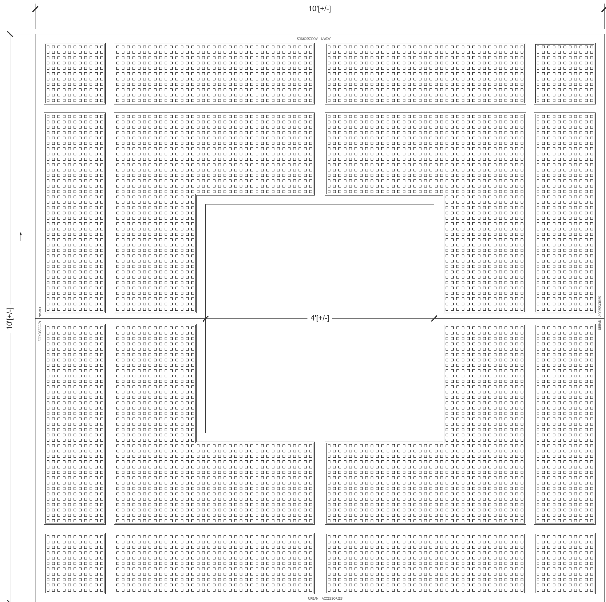
Plan Scale: 1" = 1' 0"
