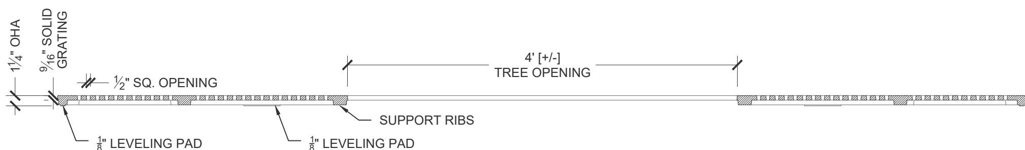
Plan Scale: 1" = 1' 0"
