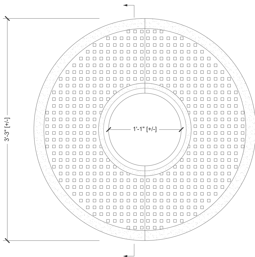
Plan Scale: 1 1/2" = 1' 0"
