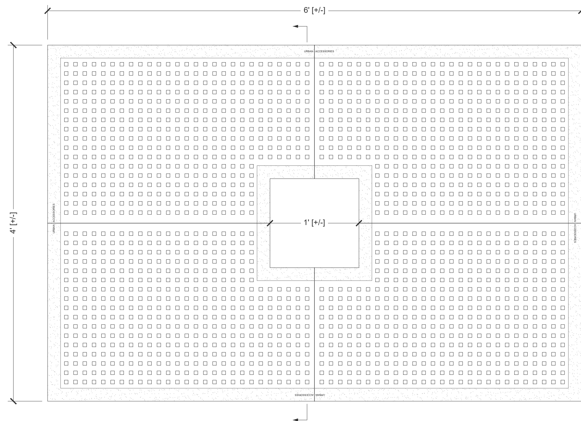
Plan Scale: 1 1/2" = 1' 0"
