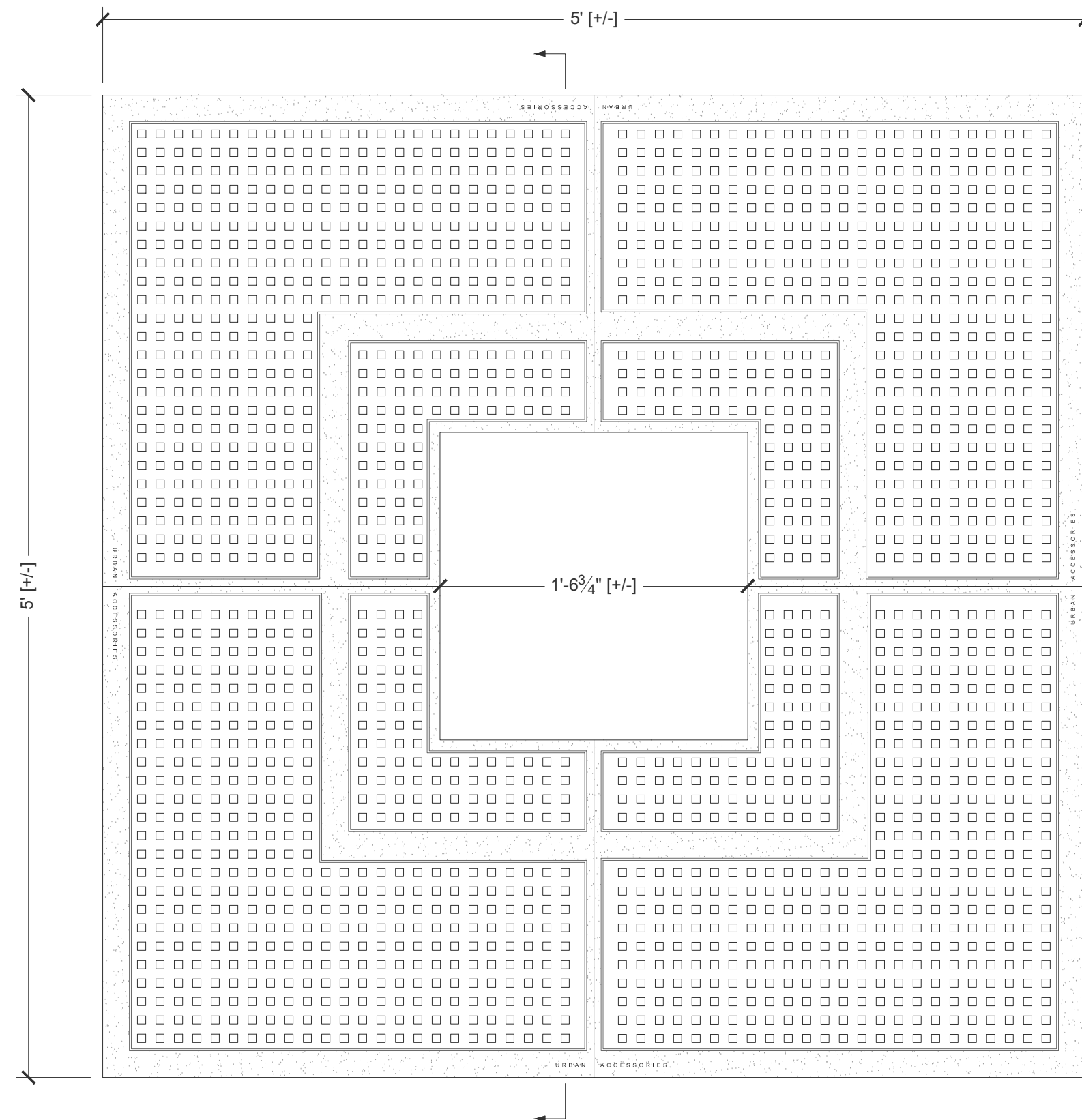
Plan Scale: 1 1/2" = 1' 0"
