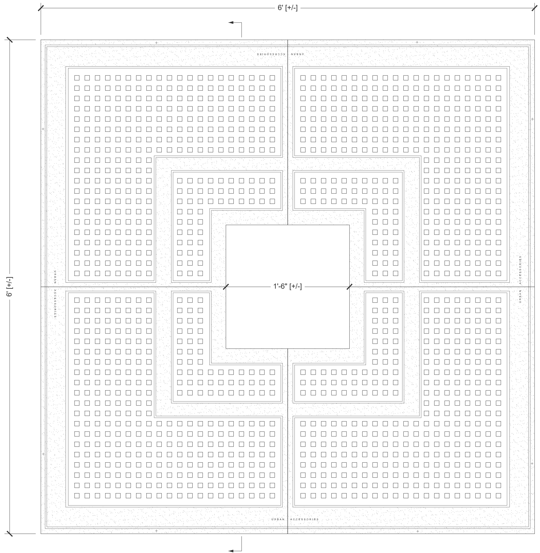
Plan Scale: 1 1/2" = 1' 0"
