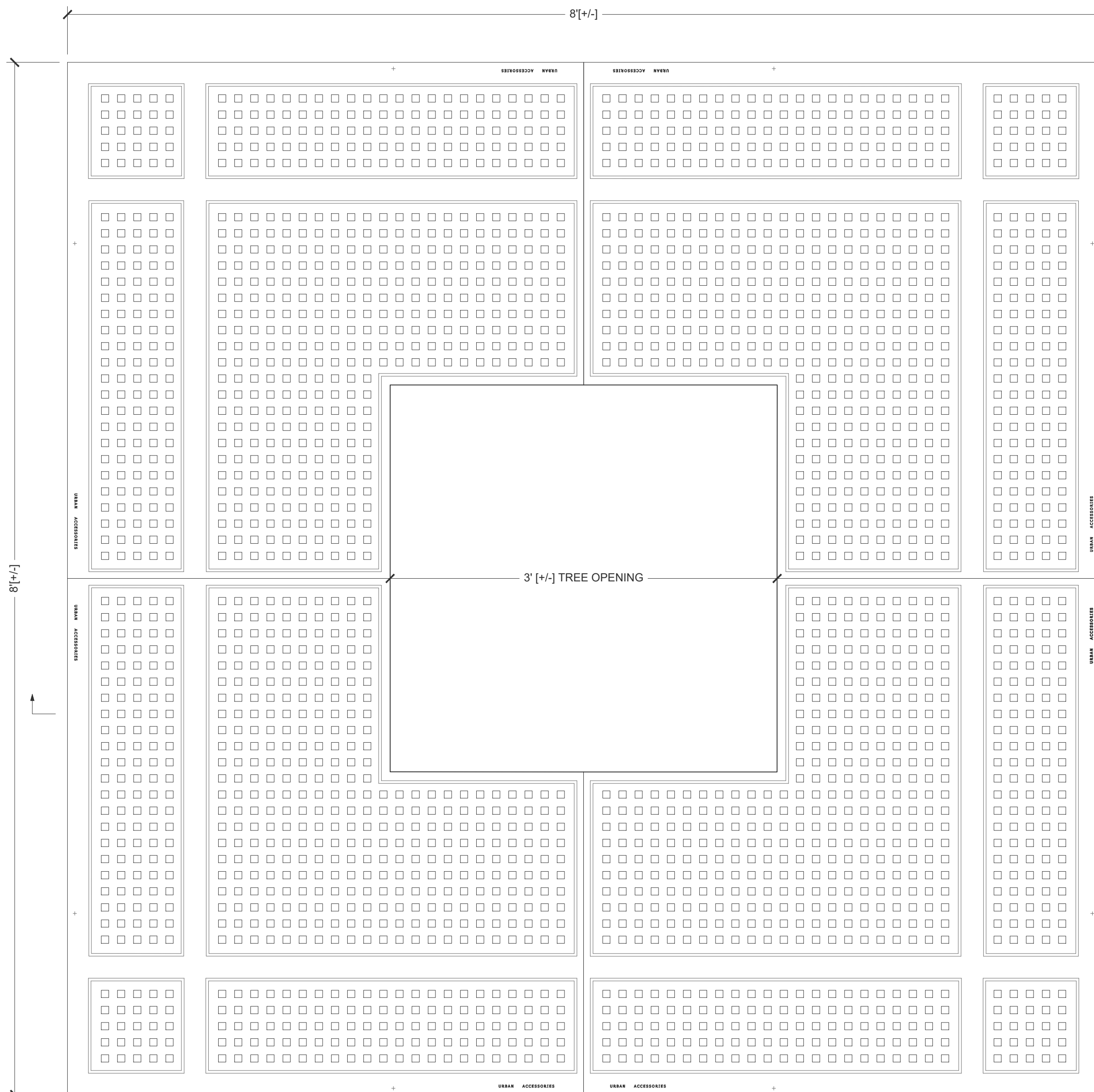
Plan Scale: 1 1/2" = 1' 0"
