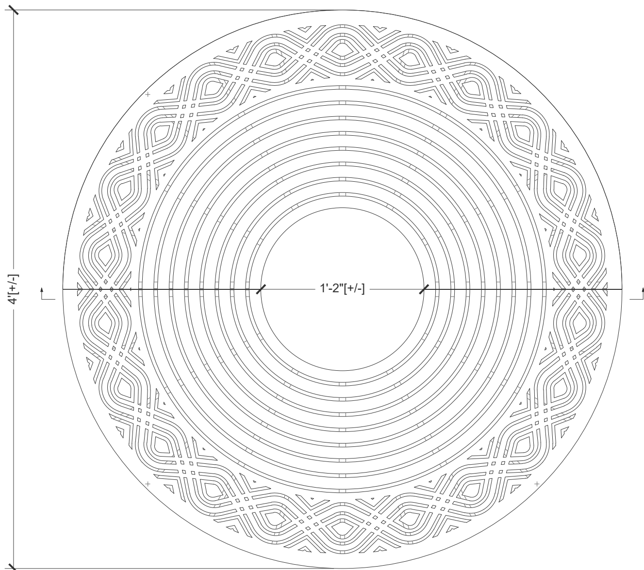
Plan Scale: 1 1/2" = 1' 0"
