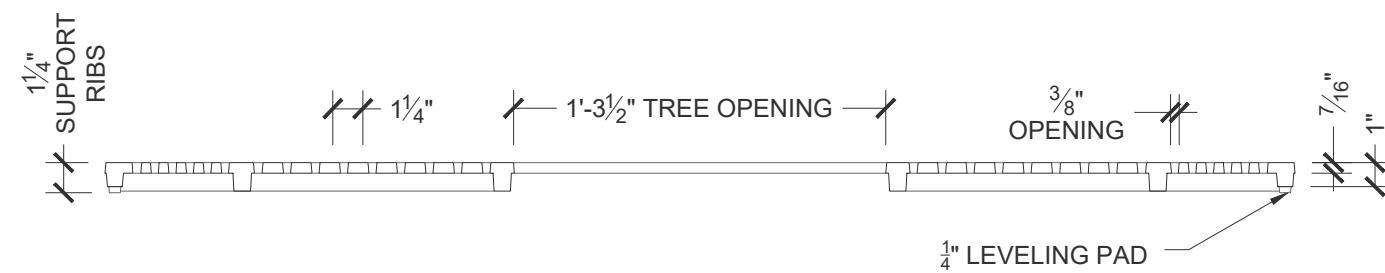
Longitudinal Section Scale: 1 1/2" = 1' 0"
