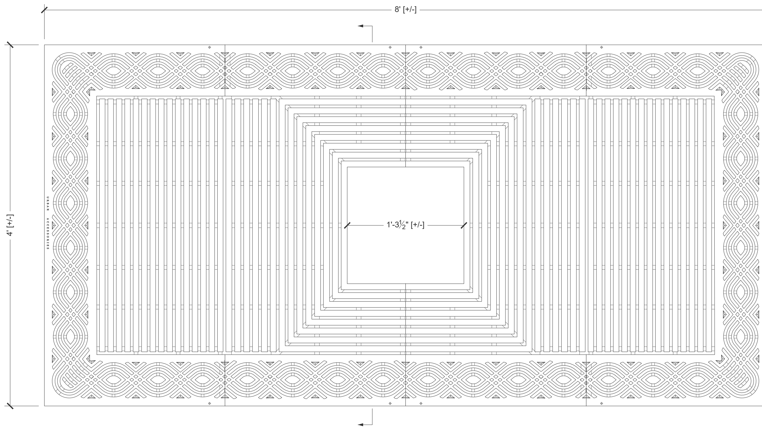
Plan Scale: 1 1/2" = 1' 0"
