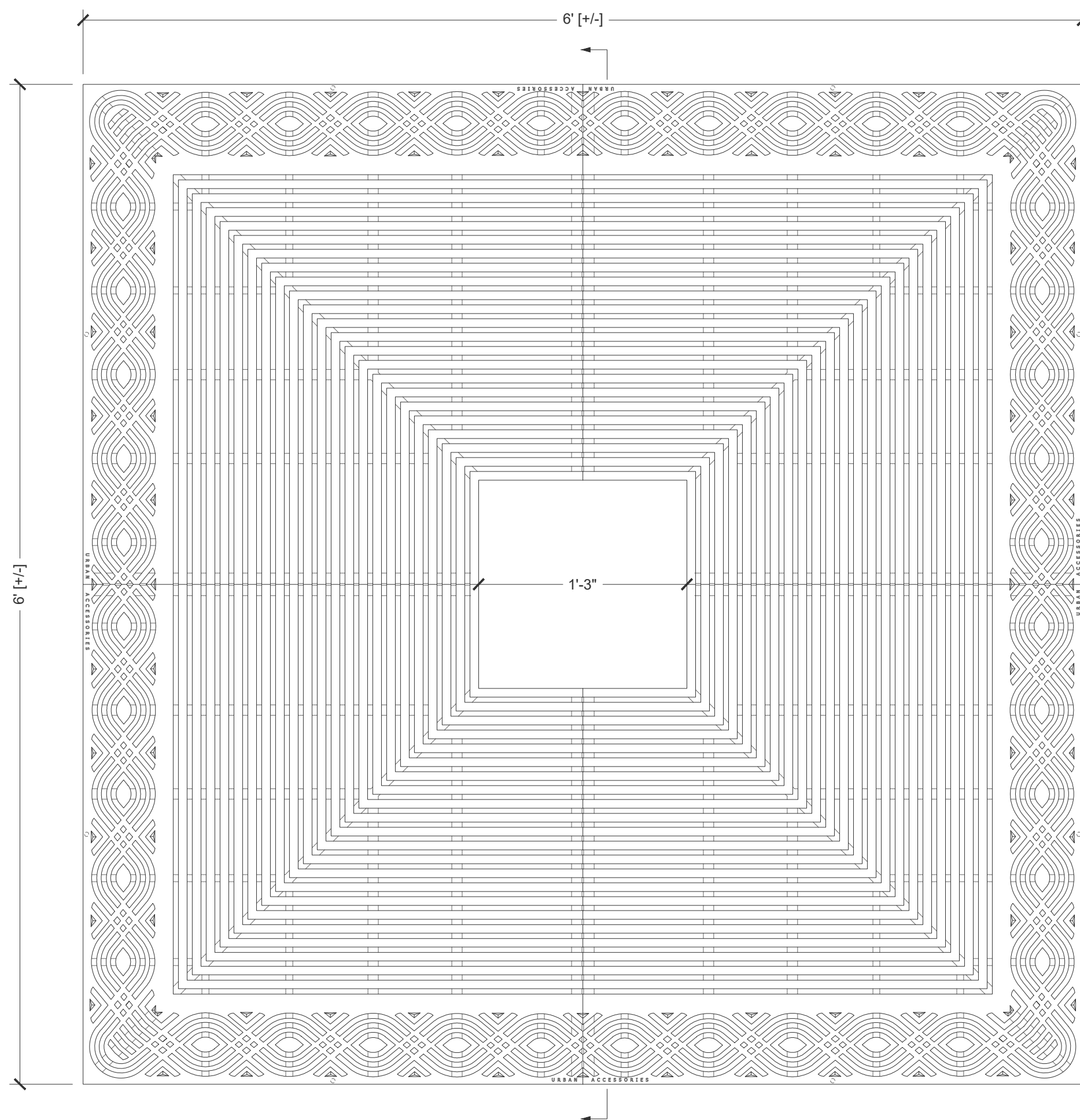
Plan Scale: 1 1/2" = 1' 0"
