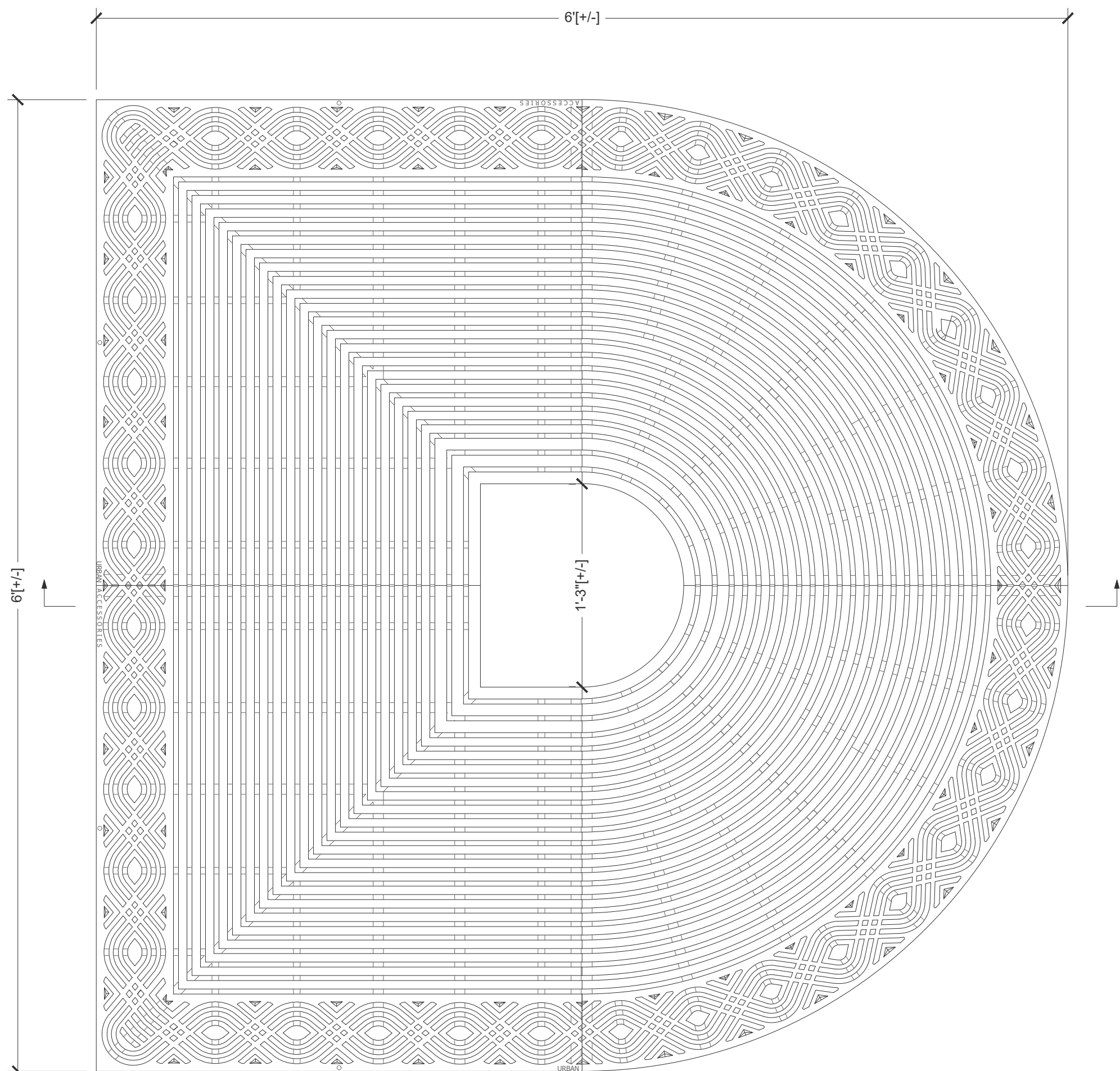
Plan Scale: 1 1/2" = 1' 0"
